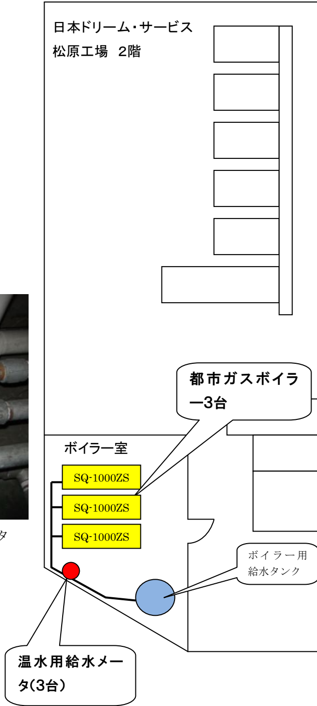
都市ガスボイラーと温水用給水メータの配置概略図
