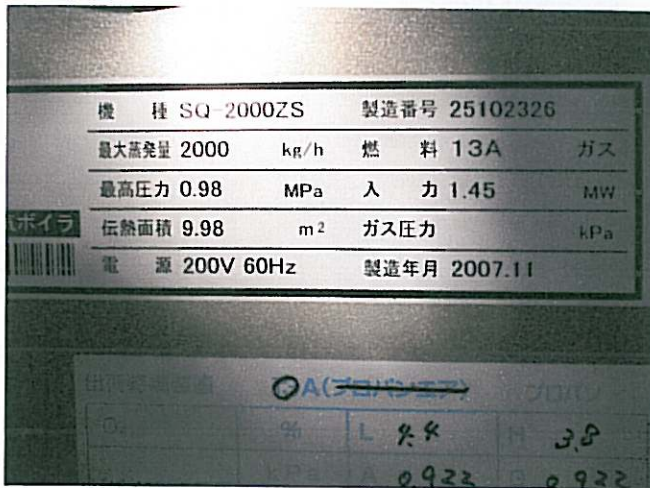
ボイラ 銘板 NO. 3
